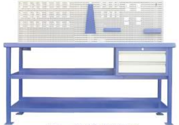
Takım Tezgâhı Sac Ortası Bölmeli 700 x 2000 mm
